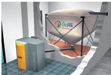
TRANSFERT PAR VIS AVEC SILO MACONNÉ OU SILO EN TOILE © ÖKOFEN
