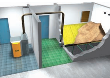
TRANSFERT PAR ASPIRATION AVEC SILO MACONNÉ OU SILO EN TOILE © ÖKOFEN
